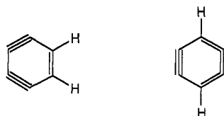
Fig. 4. 1,3- and 1,4-Benzdiyne
